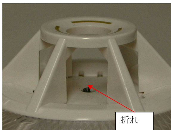
定温式スポット型感知器の損傷（サーミスタ折れ）
