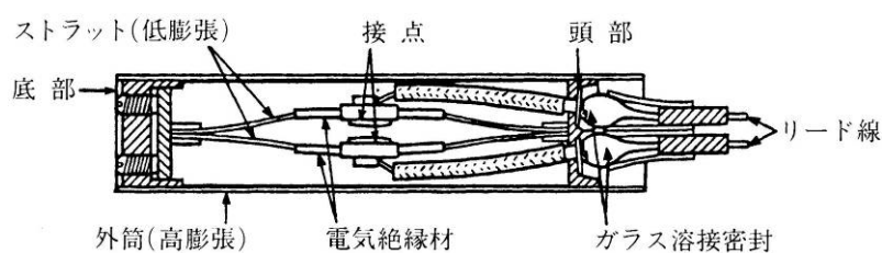
金属の膨張係数の差を利用したもの
