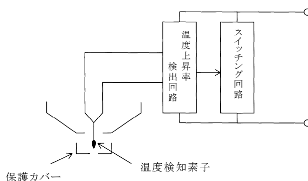
温度検知素子を利用したもの
