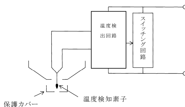
温度検知素子を利用したもの
