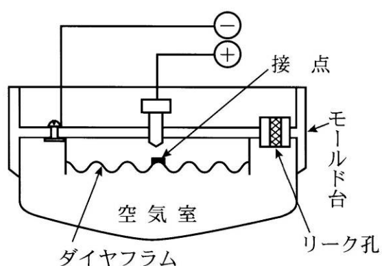
空気の膨張を利用したもの
