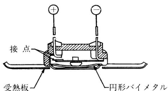
バイメタルの反転を利用したもの
